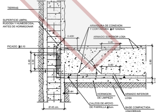
CONEXIÓN LOSA DE CIMENTACIÓN PANTALLA DE PILOTES
