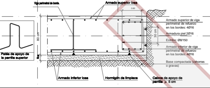
Detalle tipo de losa de cimentación
