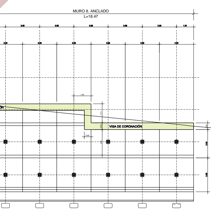
PLANTA GUÍA DE MUROS.
