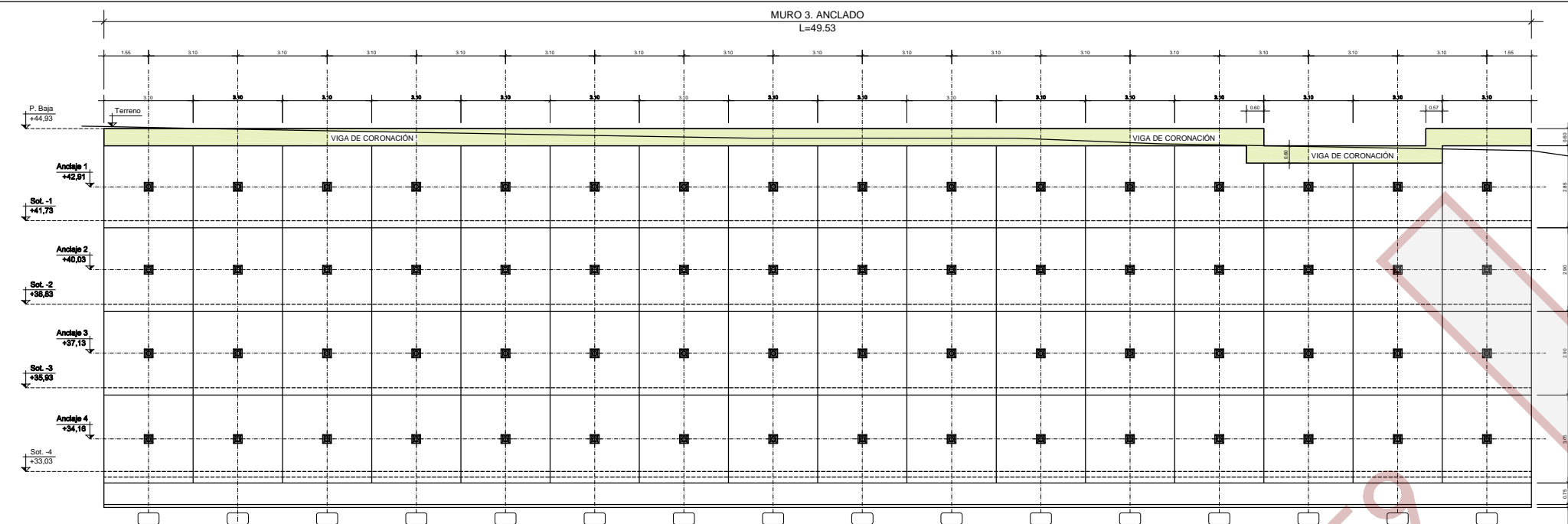
MURO 3. ESCALA: DINA A1 1:50 / DIN A3 1:25
