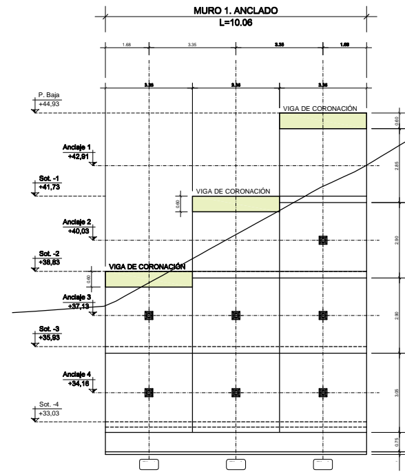
MURO 1. ESCALA: DINA A1 1:50 / DIN A3 1:25
