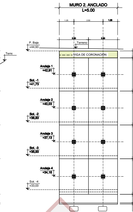
MURO 2. ESCALA: DINA A1 1:50 / DIN A3 1:25
